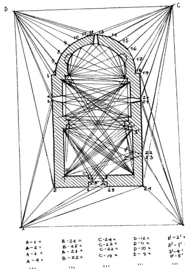
Şəkil 7. Kiş, Şəki. Məbədin plan üzrə trianqulyasiya ölçməsi
